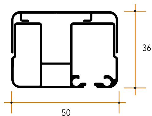
Guida telescopica Estetika motorizzata
