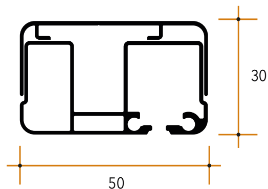
Cassonetto e barra maniglia
