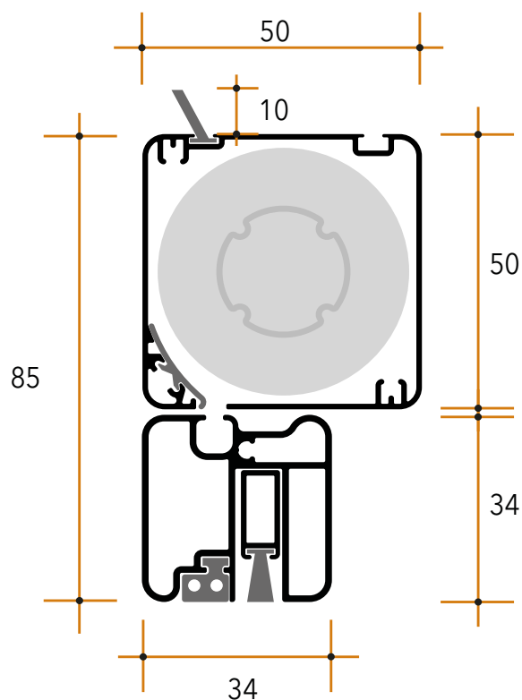
Cassonetto e barra maniglia
